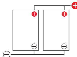
Parallelschaltung:
