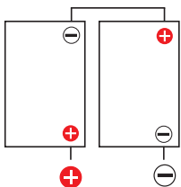
Reihenschaltung:
